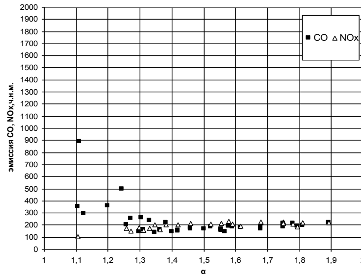
Емісія \text{CO} і \text{NO}_x при спалюванні вологої тирси ( W=49,5\% ) в глибокій реторті з решіткою допалювання
