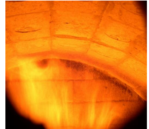
Схема глибокої реторти і фото полум'я над нею : тирса, W=45\% , q=557\text{ кВт/м}^2 ; \text{CO} = 250\text{ ppm} ; \text{NO}_x=200\text{ ppm}
